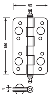
181-R INOX 304
